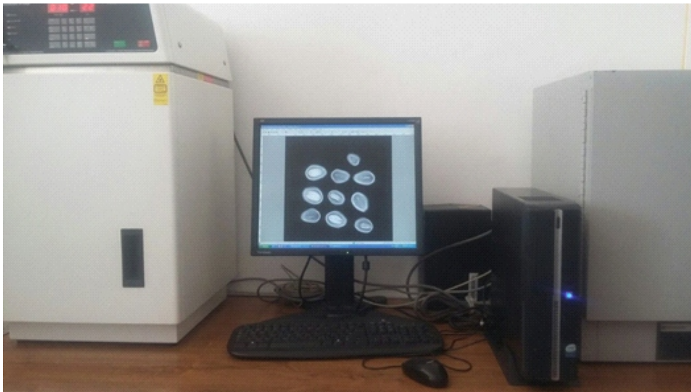
Figura 5.- Control de calidad, contraste y validación visual de la nitidez en las imágenes radiográficas obtenidas.
