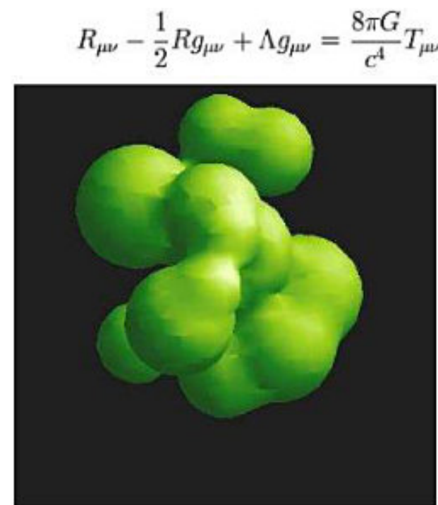
Figura.2. Representación de un universo globalmente in-homogéneo: regiones diferentes tienen tamaños y tasas de expansión distintas, dependiendo del valor inicial del inflatón. (Según Chaotic Inflation Overview).
