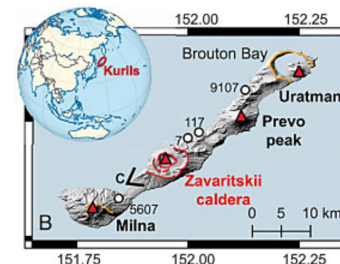
Figura 2. Mapa de ubicación de la caldera de Zavaritskii, isla Simushir, Kuriles. Detalle de la isla Simushir que muestra los volcanes, los contornos de la caldera (en naranja y rojo) y las ubicaciones de muestreo. Fuente: Modificado de Hutchison et al, (2025).
