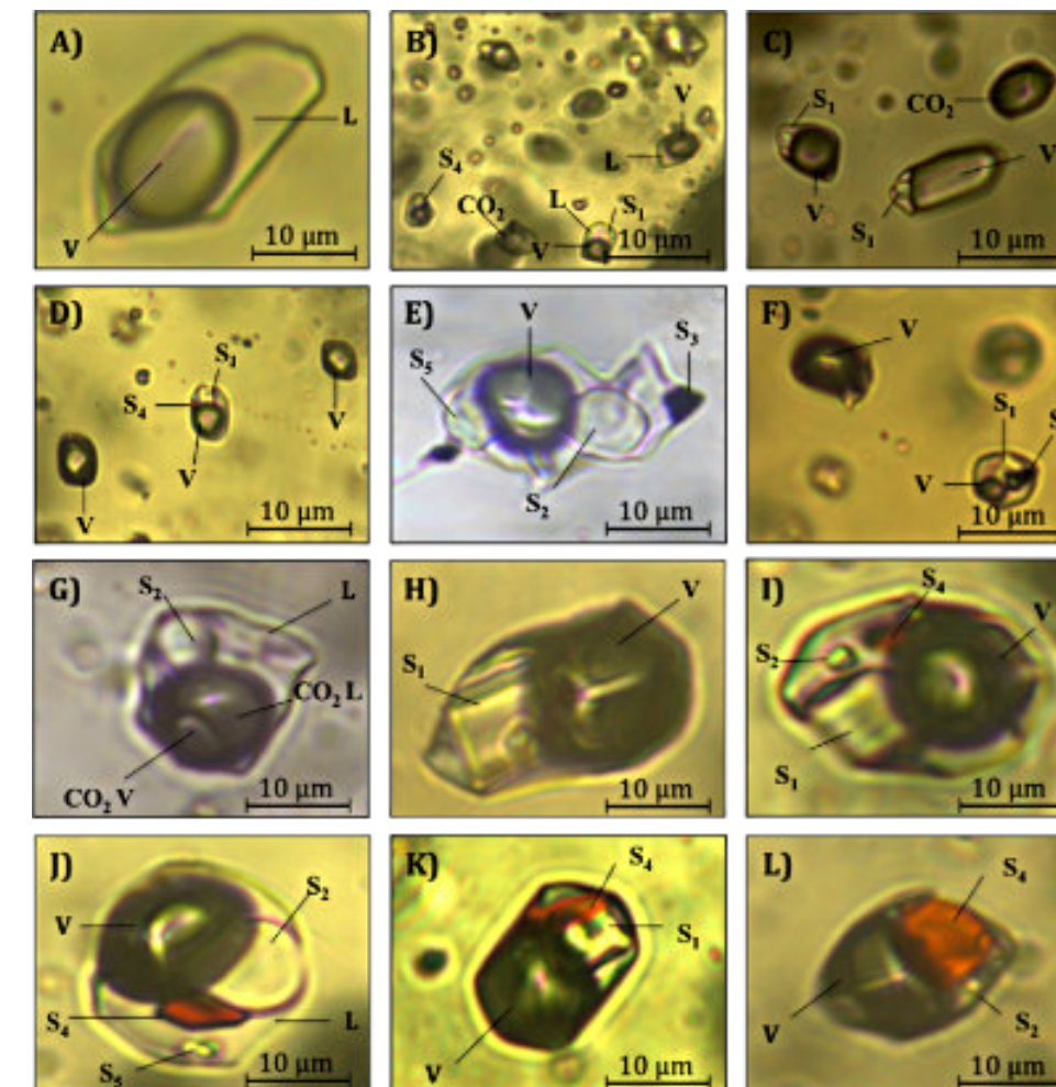
Figura # 2.- Inclusiones fluidas características de un skarn, donde el proto-fluido magmático es sub-saturado de alta temperatura (A) a L+V, para pasar a un fluido heterogéneo por ebullición (B a L) a S+L+V, con la presencia de CO 2 en fase L+V. Donde: L= fase líquida, V= vapor, S1= cubo de sal NaCl, S2= KCl, S3= Calcopirita, S4= Hematita, S5= otros complejos clorurados.
