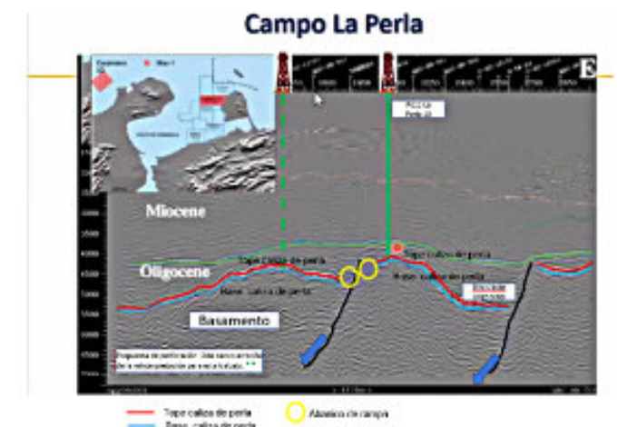
Figura 4. Reinterpretación sísmica 3D del área del Campo Perla realizada en este trabajo. Se visualiza dos bancos carbonáticos o arrecifales de geometría lenticular, acúñándose en los flancos de los paleo altos y cuñas de abanico de rampa. Se propone perforar 2º crecimiento arrecifal. Modificado de Ardila; L. Ejemplo de campos productores de arrecifes, caso Perla. Ponencia para la ACGGP 15/05/2020.
