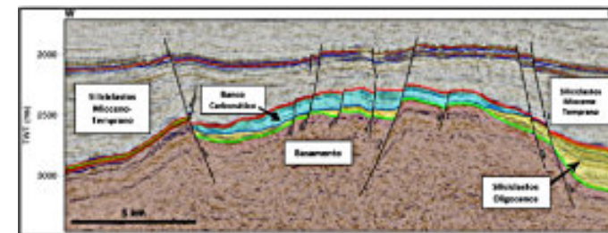
Figura 3. Imagen sísmica del banco carbonático de «Perla» (azul claro), donde se muestra su relación estratigráfica y estructural. Tomado de Palacios (2013).
